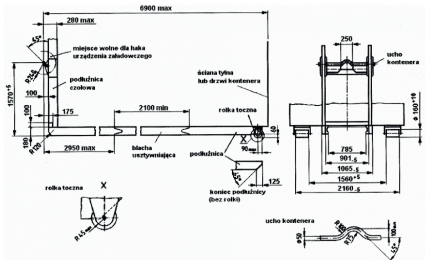
Ryc. 1. Wymiary podstawowe kontenera (gabarytowe oraz połączeniowe z urządzeniem załadownym)
