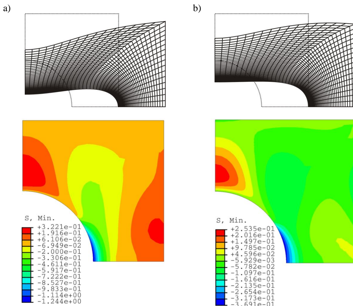
Rysunek 5.5. Deformacje siatki MES i minimalne naprężenia główne, tarcza PSN: a) zbrojona włóknami pierścieniowo, b) zbrojona włóknami promieniowo, por. rys.5.4
