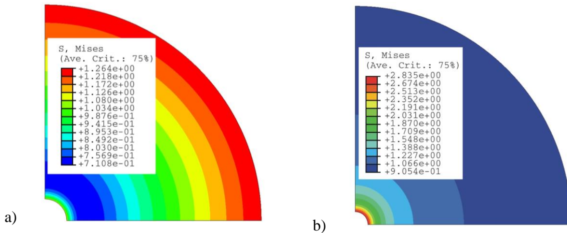
Rysunek 5.2. Wykresy warstwiczne intensywności naprężeń (naprężeń zastępczych Hubera-Misesa) uzyskane dla II siatki MES w przypadku PSN, przy zbrojeniu: a) pierścieniowym, b) promieniowym. Wyniki przeskalowane są przez q i wykonane dla r/R . Pozostałe dane są następujące: E = 2.6\mu (wyniki w naprężeniach nie są zależne od E ), \nu = 0.3 , \alpha = 0.1 , \eta = 10 , p = 0.1 . Błąd w stosunku do rozwiązania analitycznego jest mniejszy niż 1%
