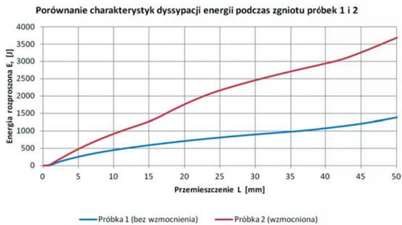
Rys. 12. Porównanie charakterystyk rozpraszania energii (dyssypacji) próbek 1 i 2
