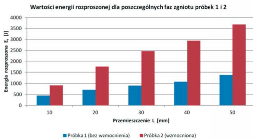
Rys. 13. Zmienność wartości rozpraszanej energii w zależności od zgniotu
