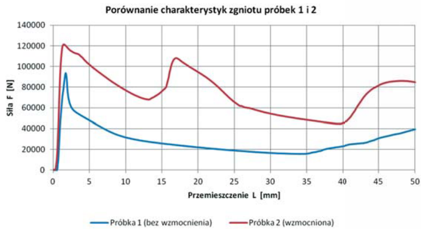
Rys.11. Porównanie charakterystyk zgniotu próbek 1 i 2
