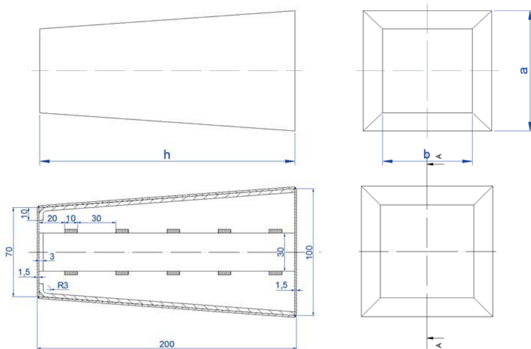
Rys. 8. Zaproponowane stalowe modele belek wzdluznych, uzyte jako próbki do badań
