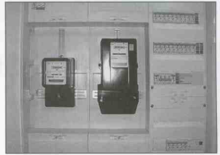
Rys. 4. Liczniki zamontowane w domu pasywnym. Jeden służy do pomiaru energii wytwarzanej przez baterie fotowoltaiczne sprzedawanej koncernowi energetycznemu. Drugi mierzy ilość energii pobranej z sieci. Zdjęcie Anna Bać
