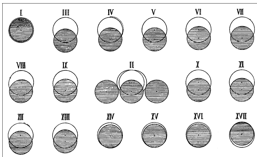
Ryc. 3. Tablica objaśniająca różne fazy zaćmienia słońca i księżyca. Ilustracja do artykułu: Uwiadomienie o zaćmieniu Księżyca i Słońca przypadającym w miesiącu kwietniu roku bieżącego , „Miesięcznik Połocki”, 1818, t. 1, nr 2, s. 133-136. Ze zbiorów BNKJ w Krakowie
