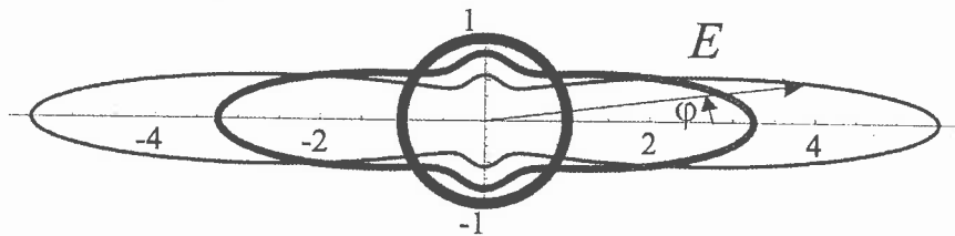
Rysunek 5.1. Wykresy modułów Younga kompozytu, o izotropowej osnowie ( \nu=1/3 ) z jedną rodziną włókien o \eta=10 , przeskalowany przez moduł Younga matrycy E(\varphi)/E : linia gruba t=0 (materiał osnowy), linia o średniej grubości t=0.25 , linia cienka t=0.5
