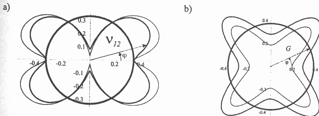
Rysunek 5.2. Wykresy: a) współczynników Poissona kompozytu \nu(\varphi) , b) modułów ścinania kompozytu G(\varphi)/E , o izotropowej osnowie ( \nu=1/3 ) z jedną rodziną włókien o parametrze \eta=10 . Linia gruba t=0 (materiał osnowy), linia o średniej grubości t=0.25 , linia cienka t=0.5
