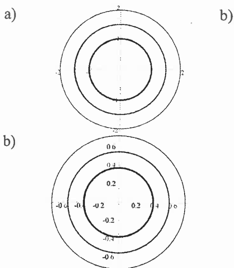
Rysunek 6.2. Wykresy: modułów Younga (a), współczynników Poissona (b) i modułów ścinania (c) kompozytu, o izotropowej osnowie ( \nu = 1/3 ) z czterema jednakowymi rodzinami włókien o \eta = 10 , które przecinają się pod kątem \pi/4 . Na wykresach (a-c), linie oznaczają: linia gruba t = 0 , linia o średniej grubości t = 0.05 , linia cienka t = 0.1 (skalowanie jw.)
